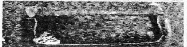
UNO MILLE FIRE FLEX - HCQ 1046 - CHASSI OXIDADO
