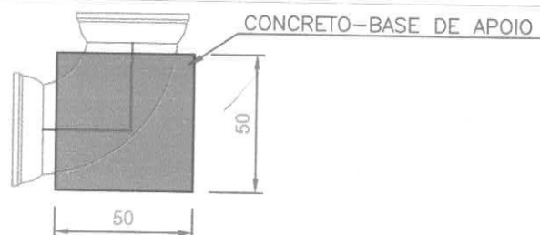
CO DE ANCORAGEM - CURVAS CORTE LONGITUDINAL
