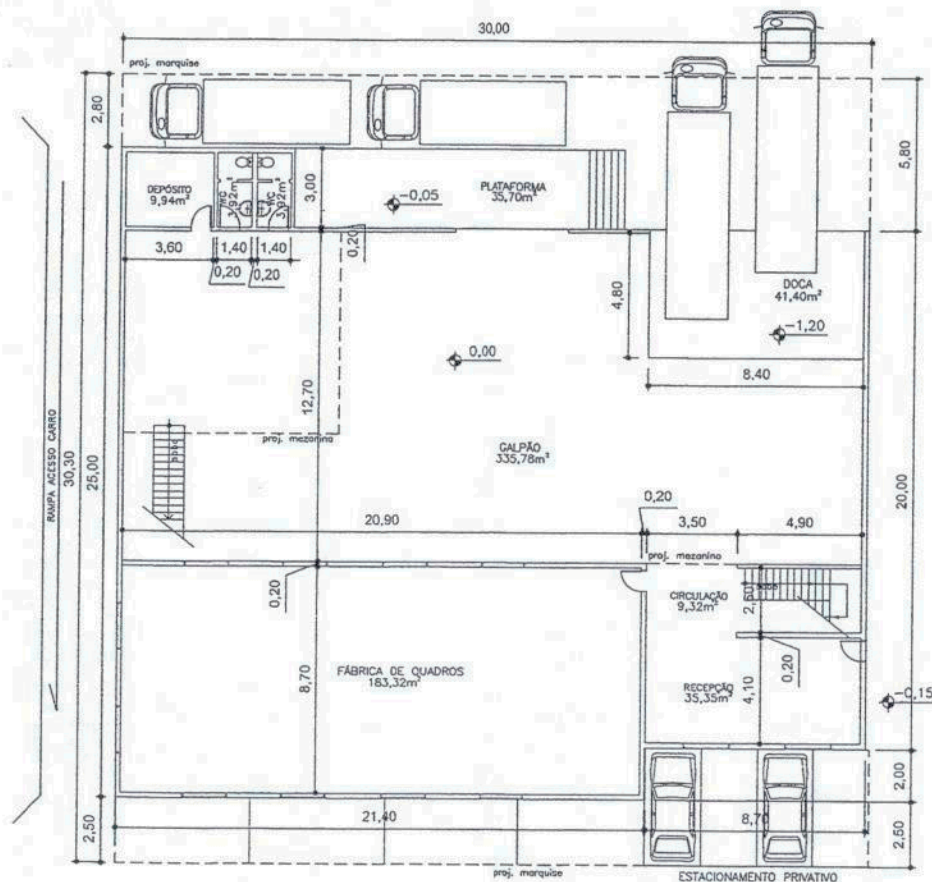
PLANTA - PAV. TERREO 658,65m² ESCALA 1:100
