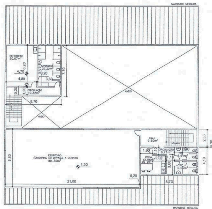
PLANTA - PAV. SUPERIOR 289,61m² ESCALA 1:100
